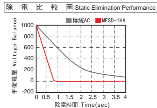
測試條件 距離 30cm Test Conditions Distance 30cm ±1000V到±100V消除靜電所需時間 Elimination time : From ±1000V to ±100V 使用150mm x 150mm CPM (20pF) Use 150mm x 150mm (20pF) CPM device
