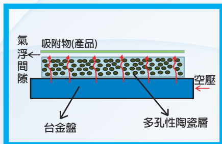
陶瓷氣浮圖示
